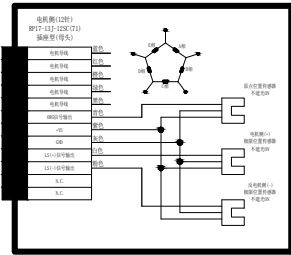
PHLP60-30X-M5接线图
