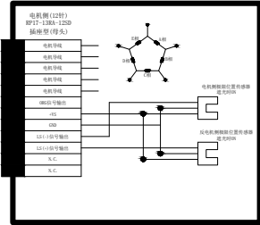
PHTM-40A40R接线图
