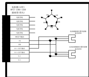
PHTM-60A105接线图
