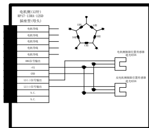
PHTM-60A85接线图
