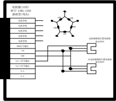
PHTM-40B60R接线图
