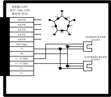
PHTM-40B40R接线图
