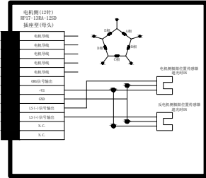
PHTM-40A75R接线图
