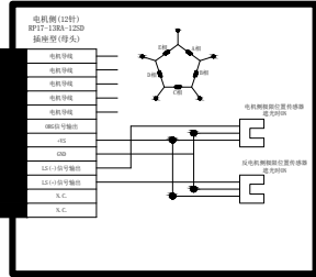
PHTM-40A75接线图
