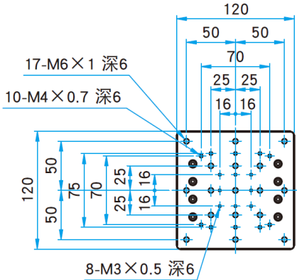
〈上板安装孔示意图〉
